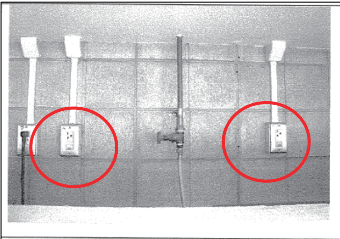
③200V 電源↑
